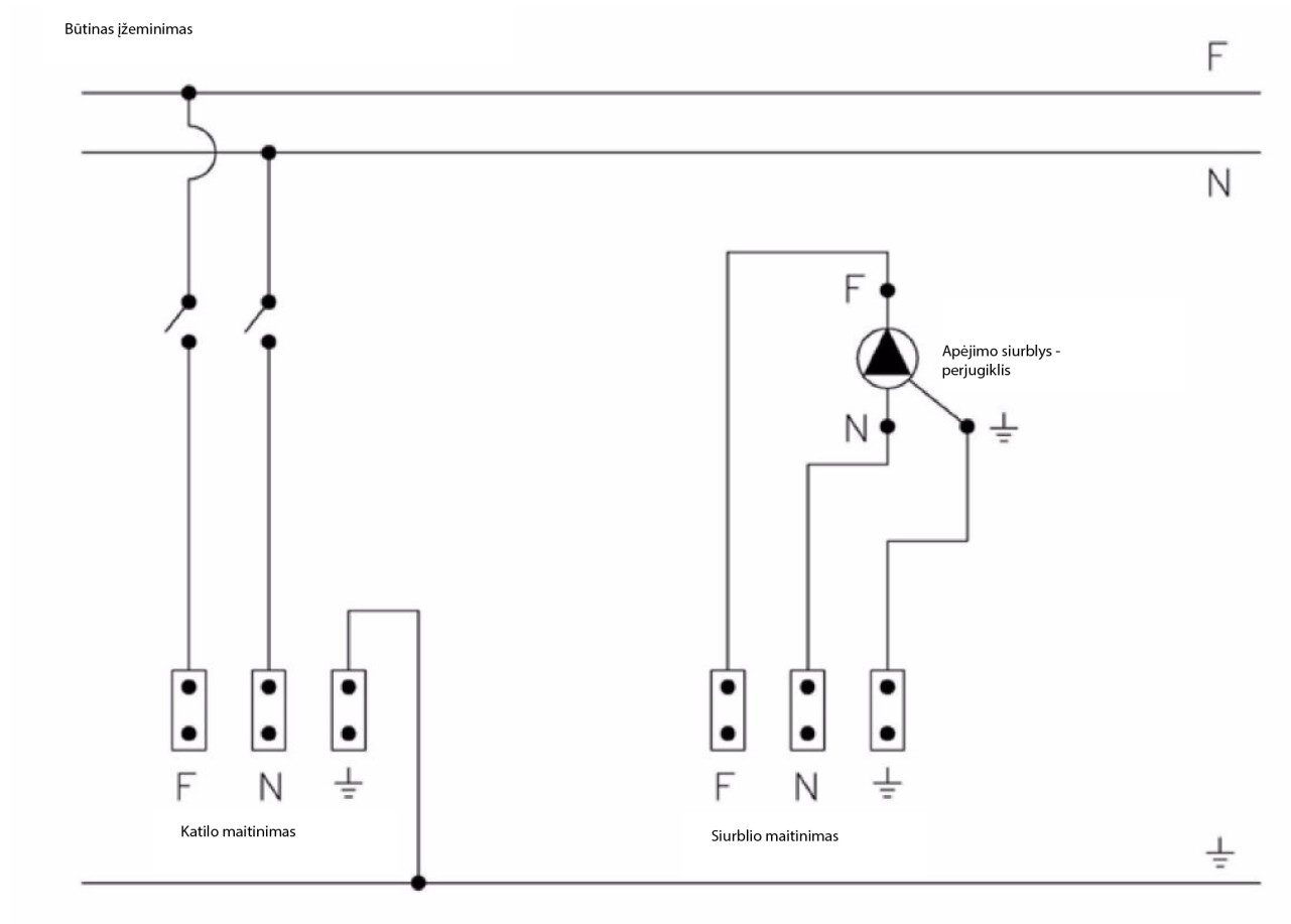
Elektros schema 3
