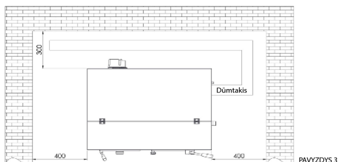
1 pav. Minimalus atstumas tarp katilo ir katilinės sienų
