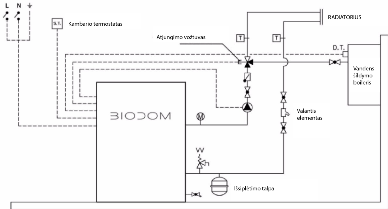
Prijungimo schema 2
