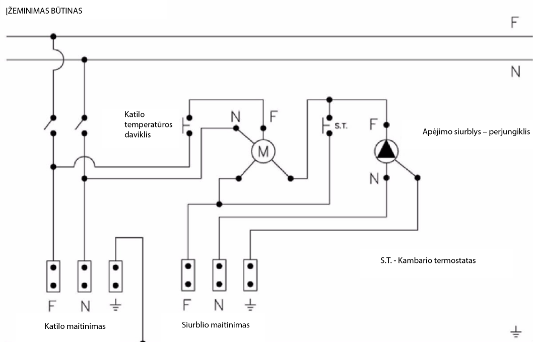
Elektros schema 2
